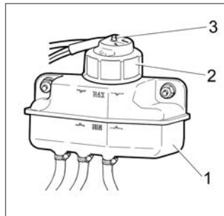
Рис. 34. Бачок гидропривода тормозов и сцепления
