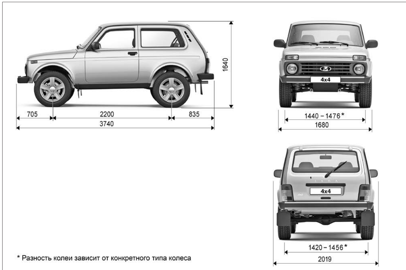
Рис. 50. Габаритные размеры автомобиля LADA 4x4 3 дв.
