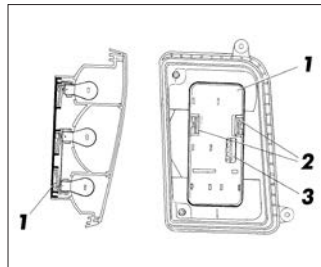
Рис. 44. Задний фонарь
