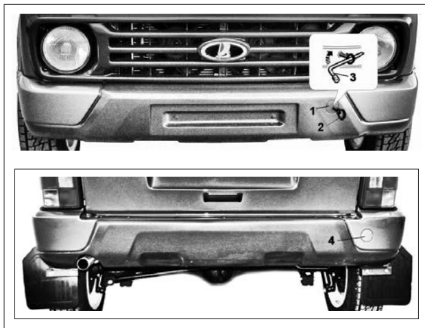
Рис. 31. Место установки буксировочной проушины
