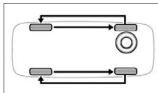
Рис. 39. Схема перестановки колес
