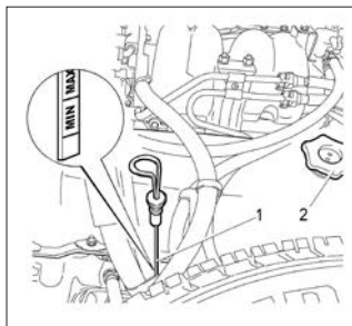
Рис. 32. Проверка уровня масла в картере двигателя
