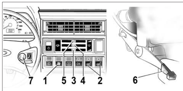
Рис. 24. Органы управления климатической установкой
