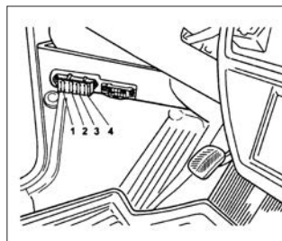
Рис. 49. Дополнительные предохранители
