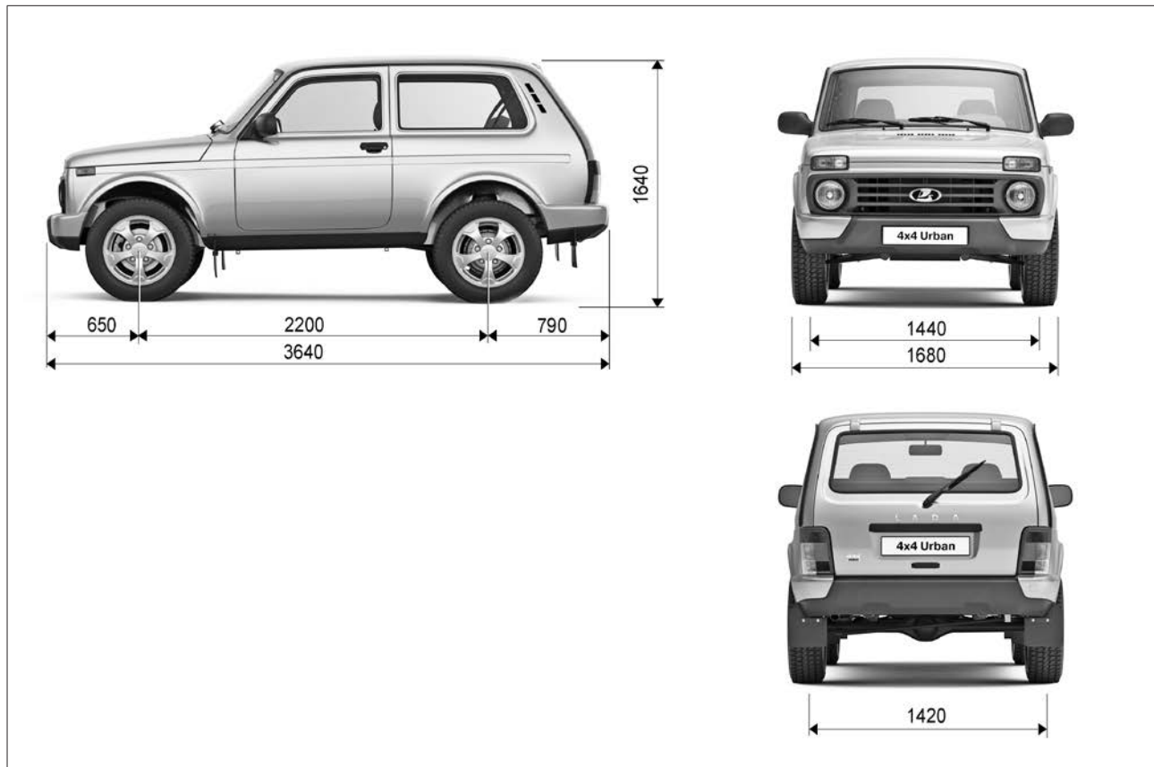
Рис.52. Габаритные размеры автомобиля LADA 4x4 Urban 3 дв.
